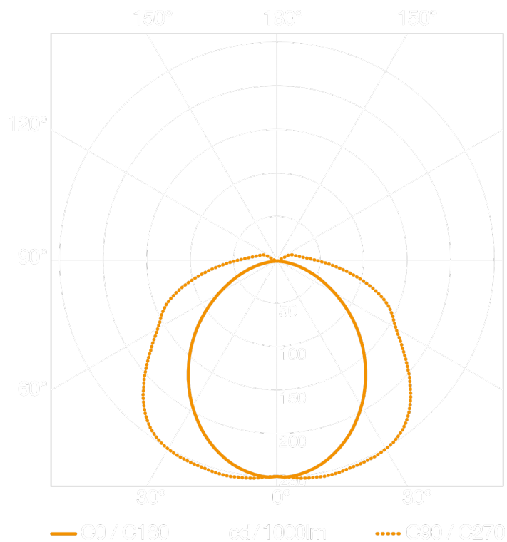
Lichtverteilungskurve 1
