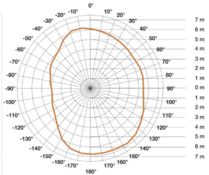
Sensorenerfassungsbereich 1
